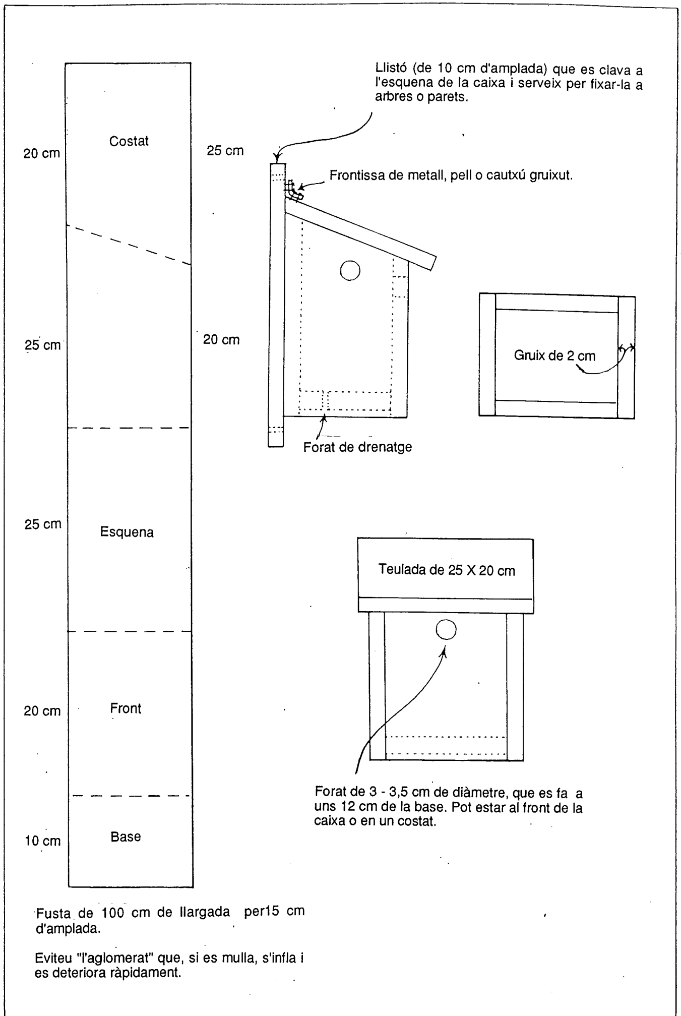
5(1). Detalls de construcció d'una caixa niu per a mallerengues (del llibre The bird table book de T. Soper)
